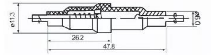
F103-C 6X30 FUSE HOLDER:
