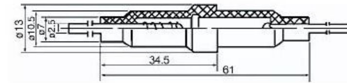
F103-C 6X30 FUSE HOLDER:
