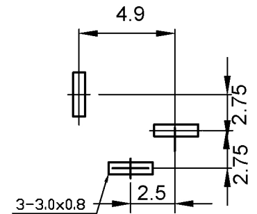
线路板安装尺寸示意图
