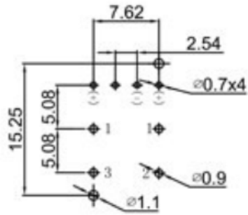
PCB开孔尺寸
