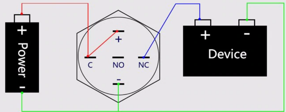
Wiring diagram 4 :
