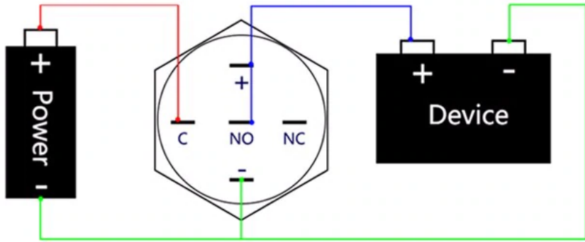
Wiring diagram 1 :
