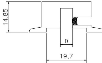
SECTION D-D
