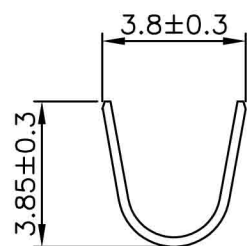
A-A SEC
