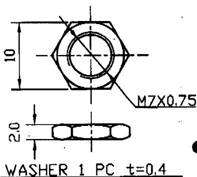
NUT 1 PC
