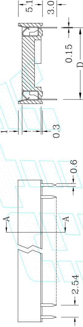
Section A-A
