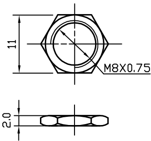
NUT 1 PC
