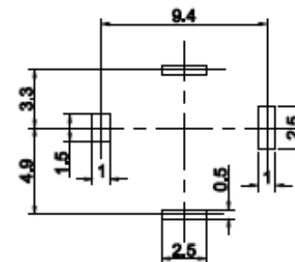
线路板印刷开孔尺寸
